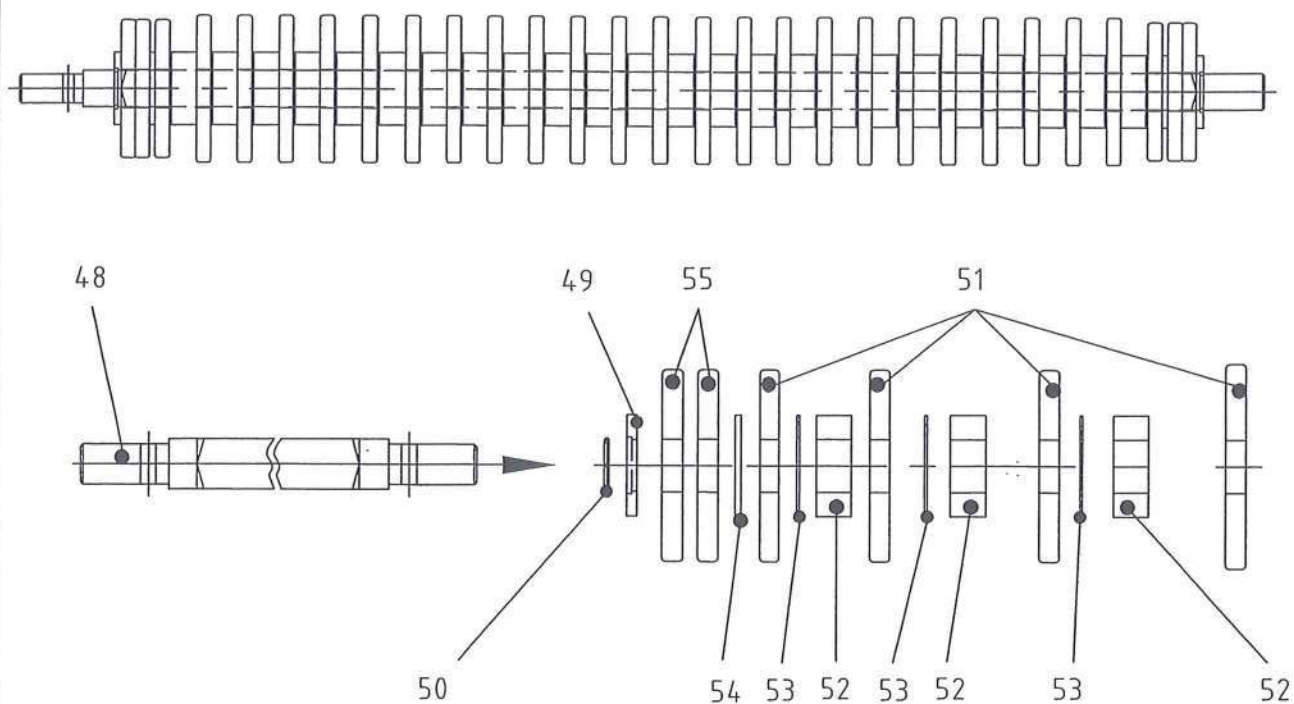
Tambour de calibrage 15mm
