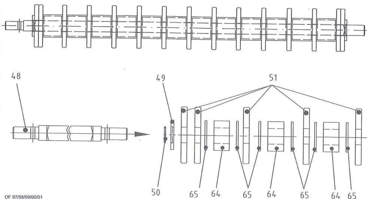
Tambour de calibrage 40mm
