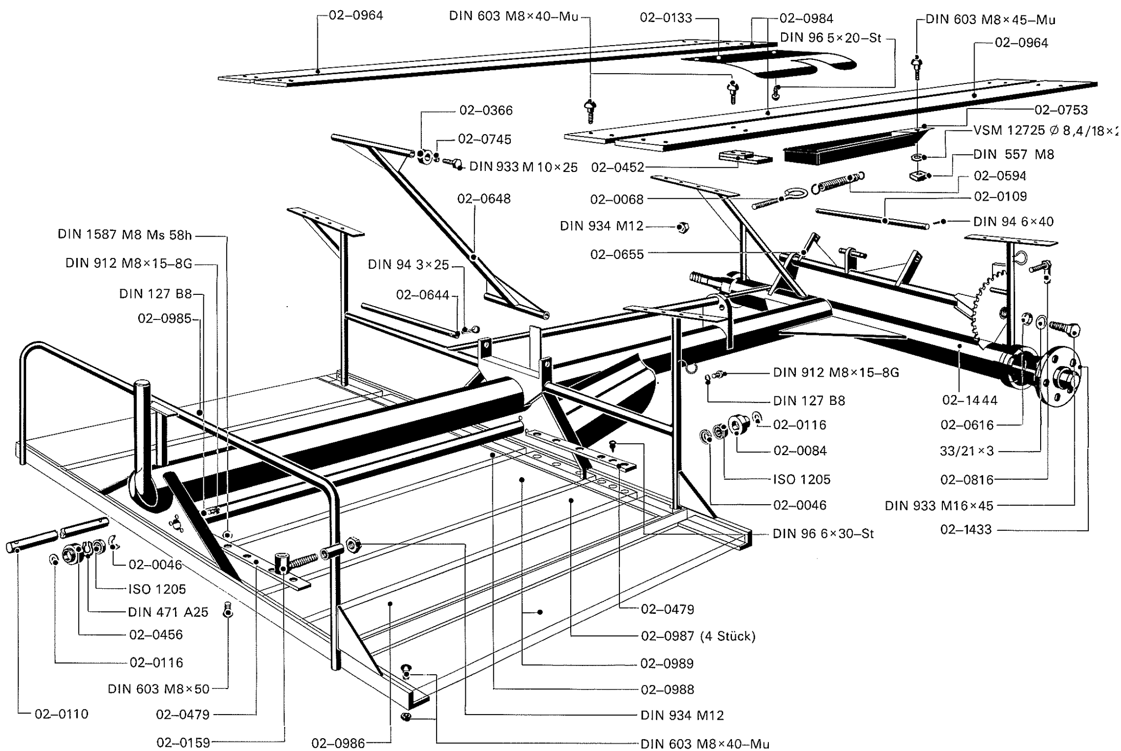
Fahrgestell für neue Fahrachse
