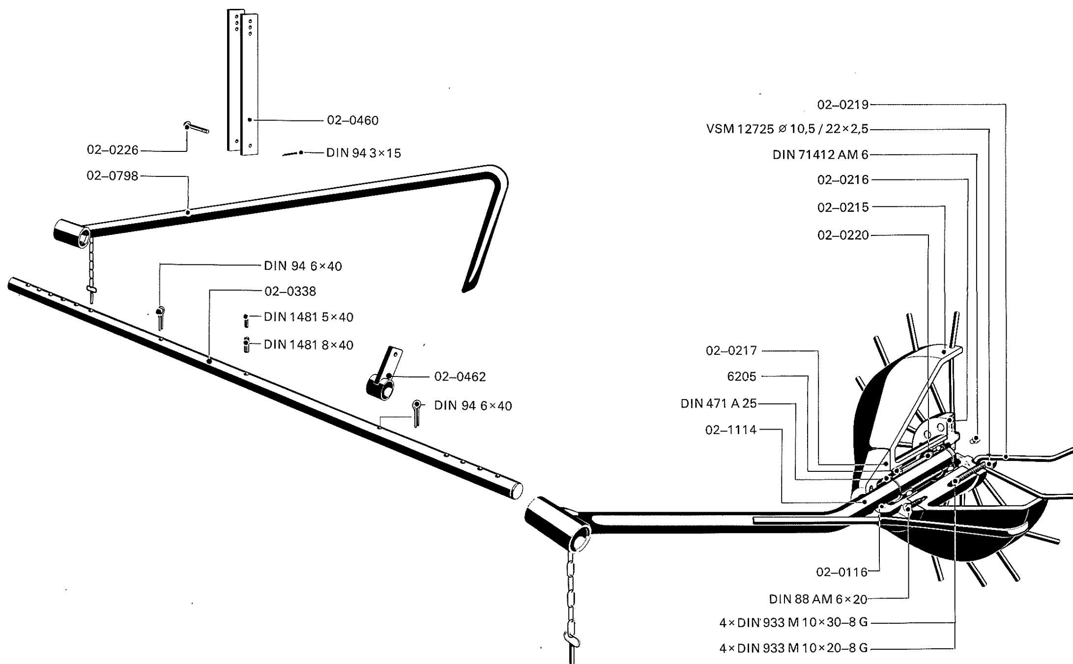
Furchenreiniger normal
