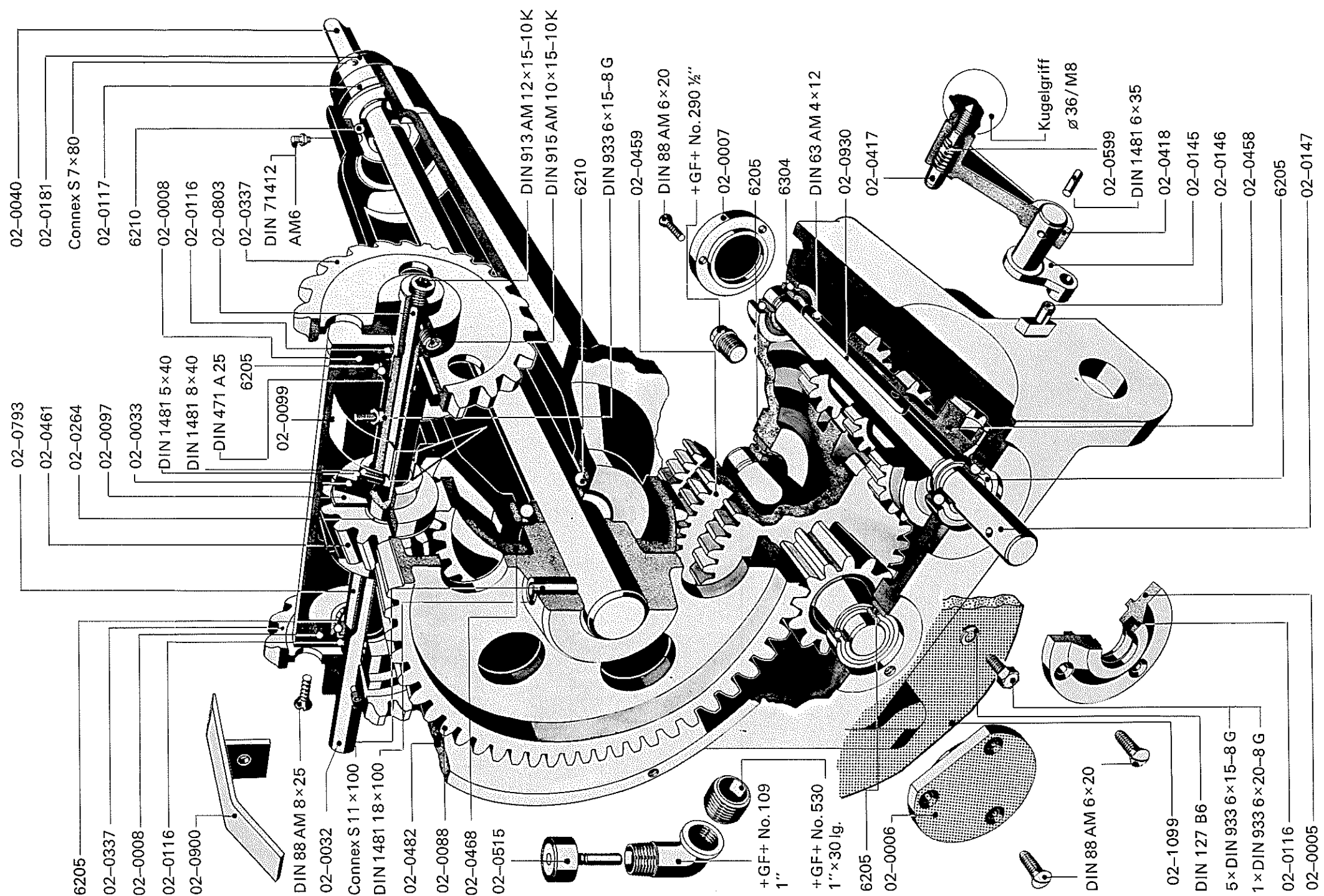
Dreiganggetriebe mit altem Getriebedeckel
