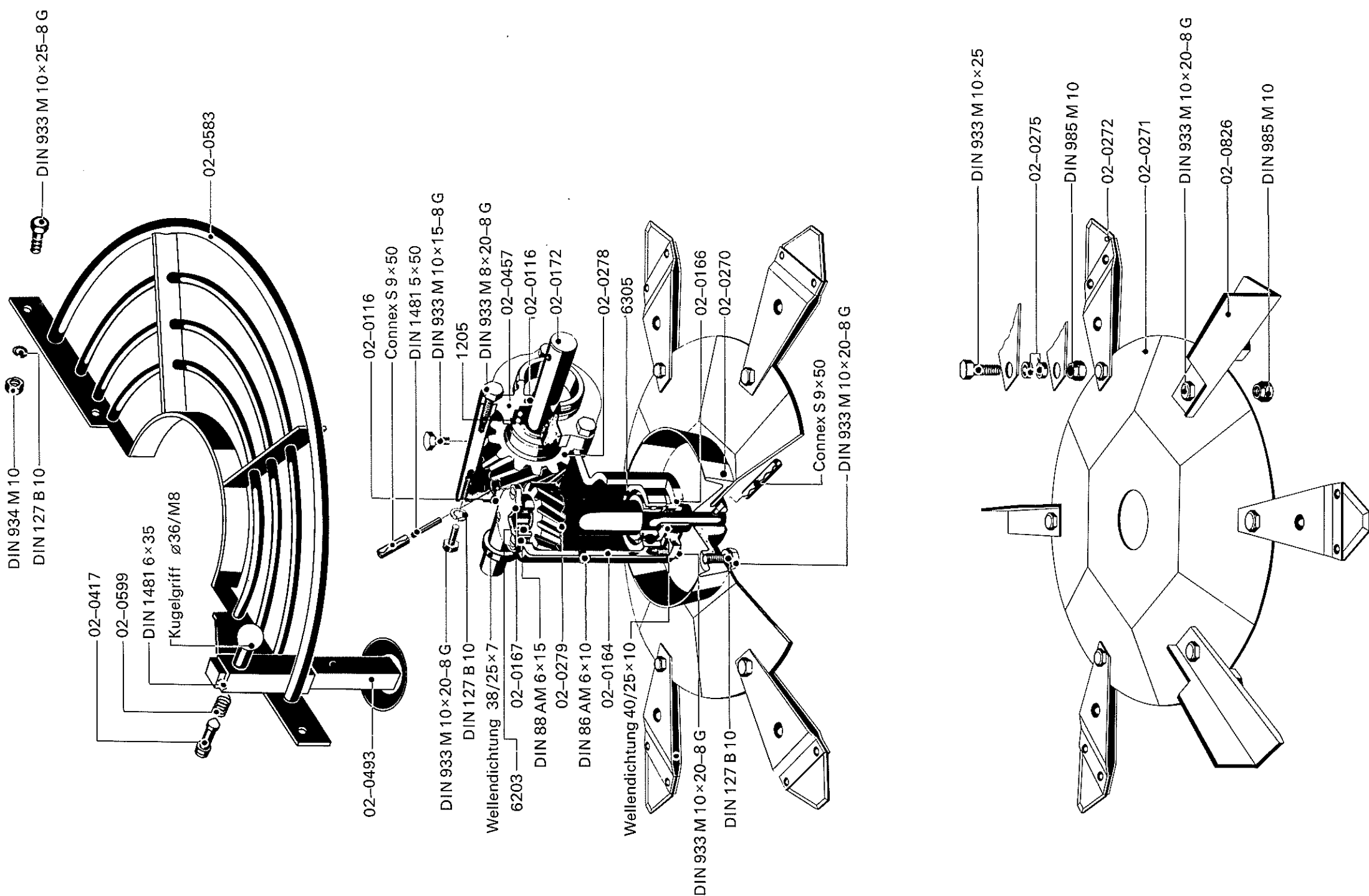
Krautschneider normal
