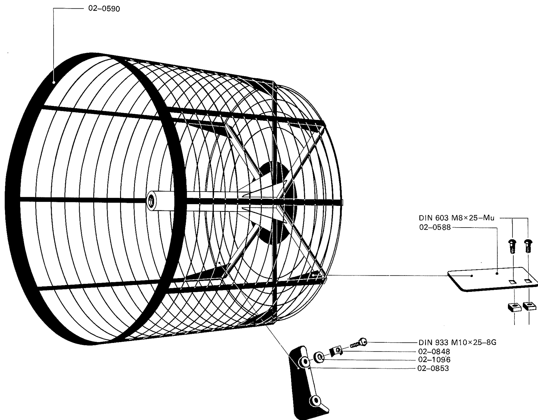
Siebtrommel für Zuckerrüben
