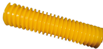
SPIRALWALZE GELB, PU LI+RE / Ø98 mm x 400 mm / 40 mm x 40 mm, mit Endscheibe
